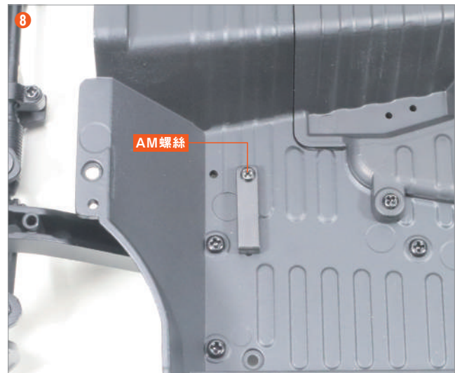
使用 AM螺絲 進行固定。
