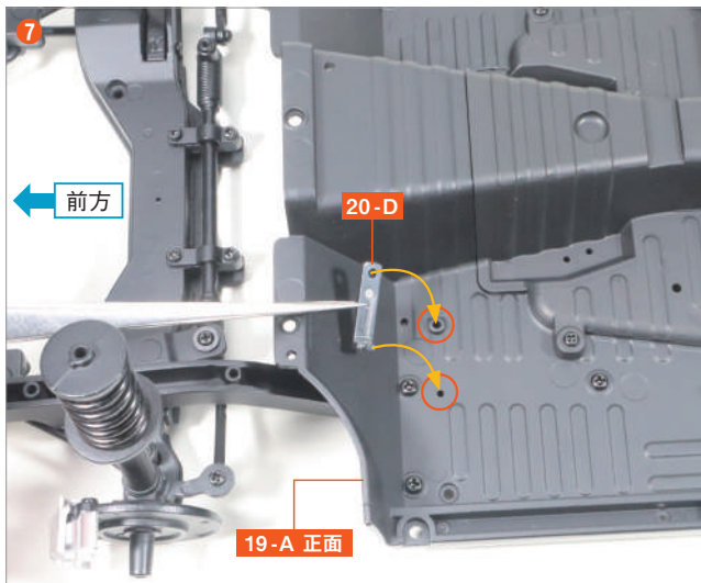
將線夾 20-D 的突起部分，對齊 19-A 的螺絲洞孔插入。
